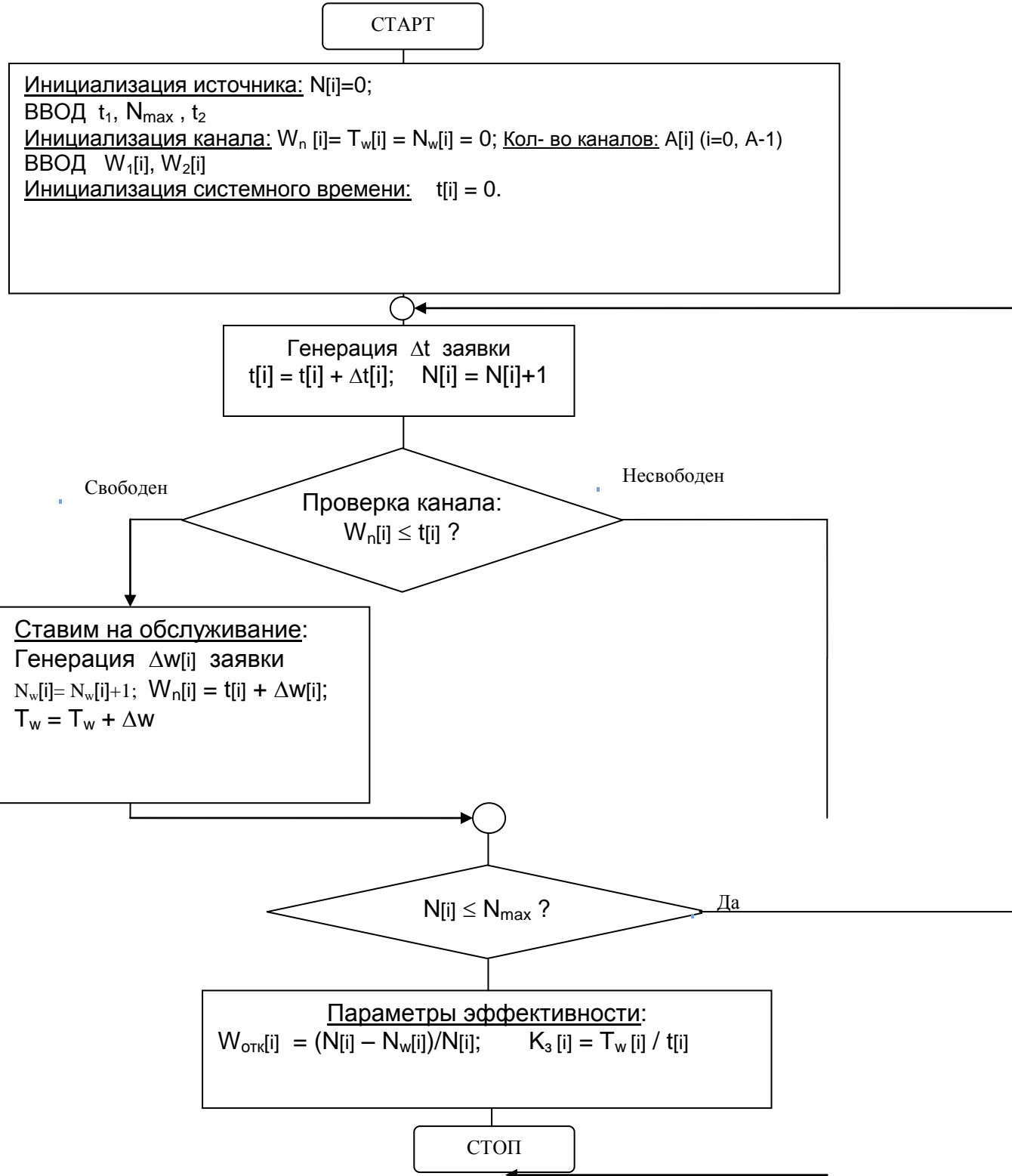
Рис.9.Блок схема одноканальной СМО с неограниченной очередью
