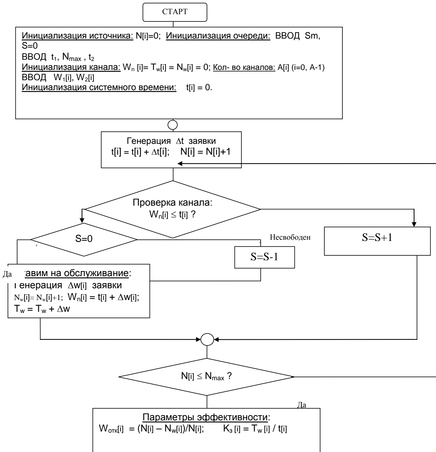
Рис.13.Блок схема n-канальной СМО с неограниченной очередью
