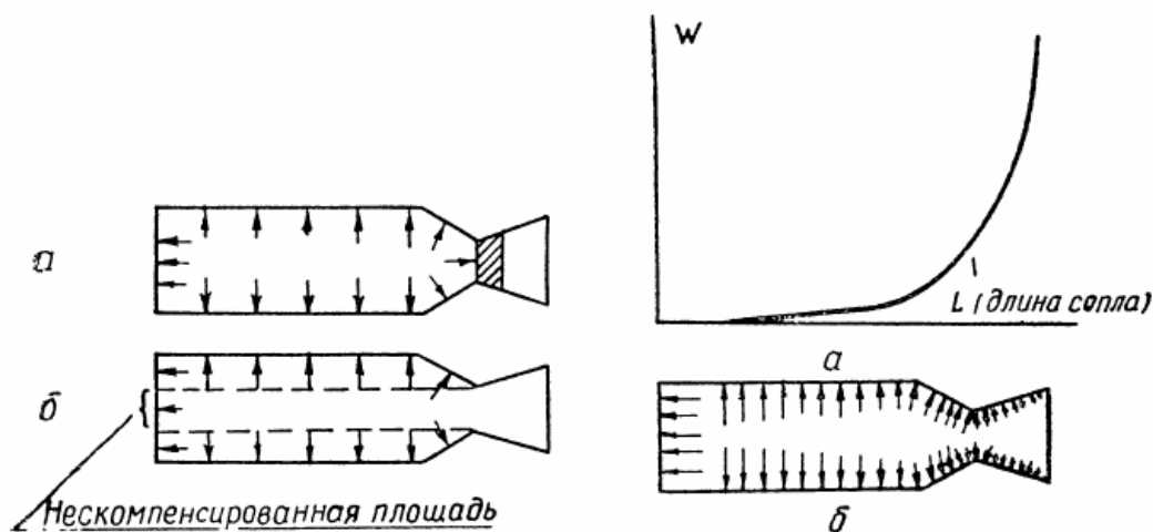
Рис. 11. Схема образования реактивной тяги в ракетном двигателе
