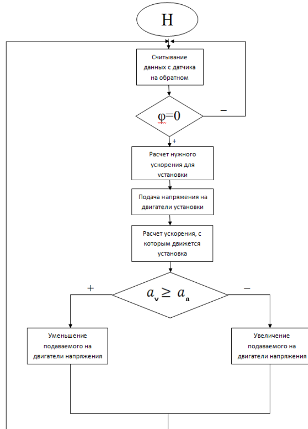
Схема №1 Блок схема работы программы управления
